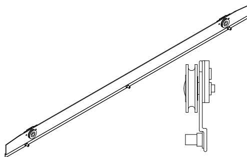
A3618, Roller Bar
