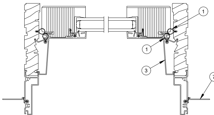
Jamb
