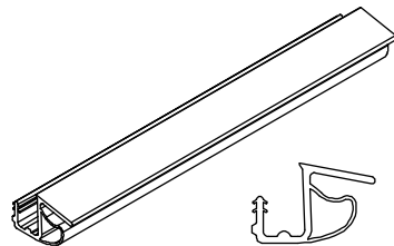
V2037, Door Sweep/Drip Beige or Black
