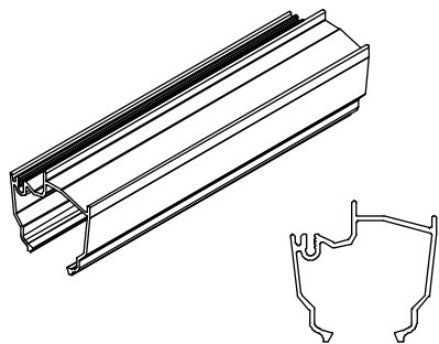
Astragal, A2047
