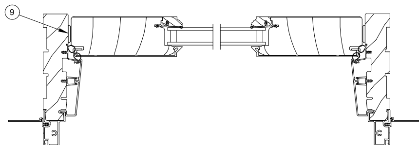
Jamb
