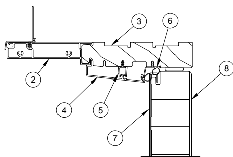
6 9/16" Jambs
