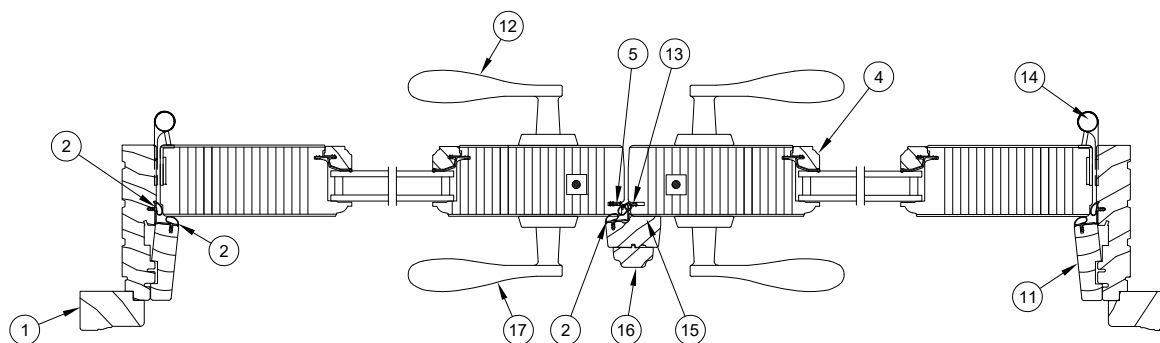
Wood Jamb Detail XX L
