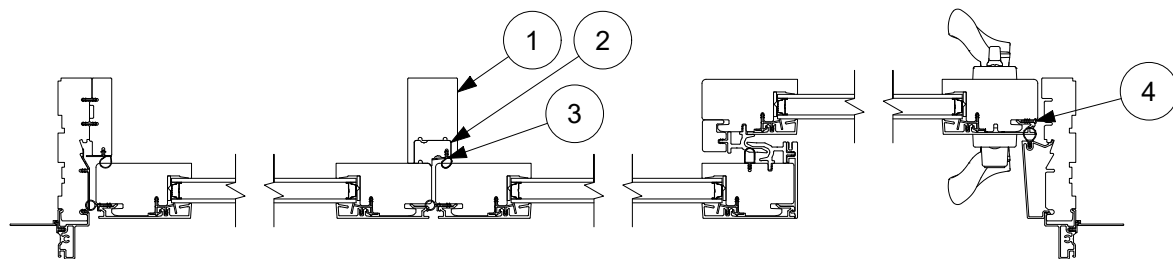
OOX - 4 9/16" Jamb - 1 3/4" Panel
