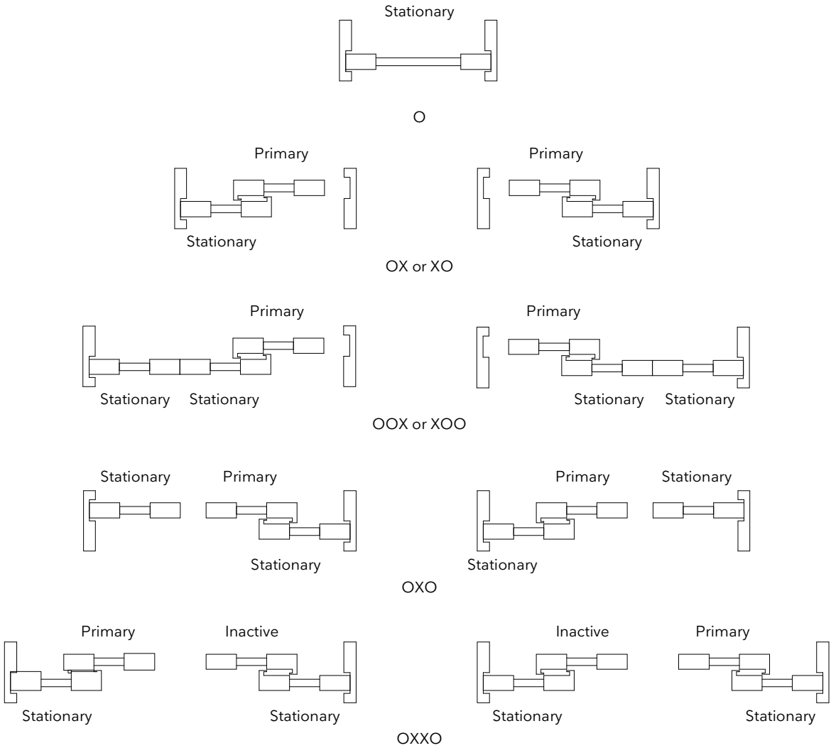
Modern Sliding Door: MSD
