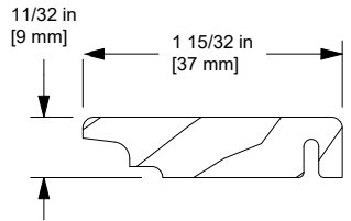
Head Jamb Stop, W10231
