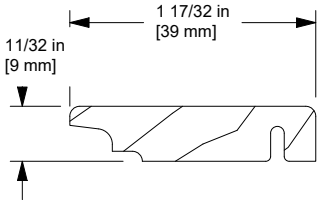
Jamb Stop, W10230
