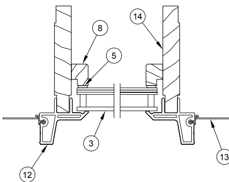
Jamb Detail
