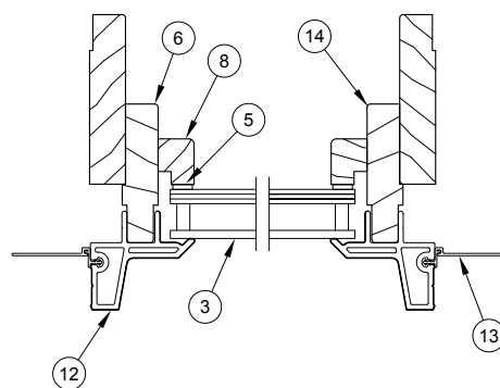
Jamb Detail
