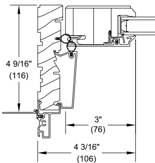
6 9/16" Sidelite Jamb
