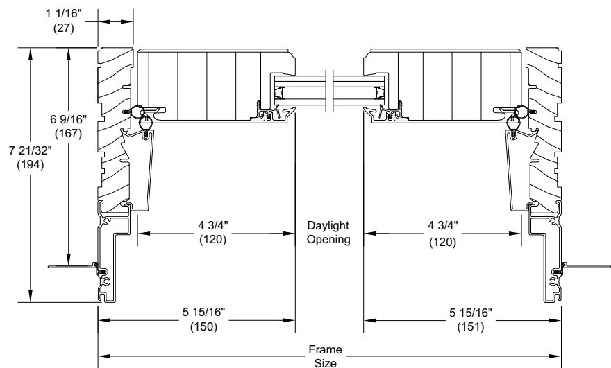
6 9/16" O - Jamb
