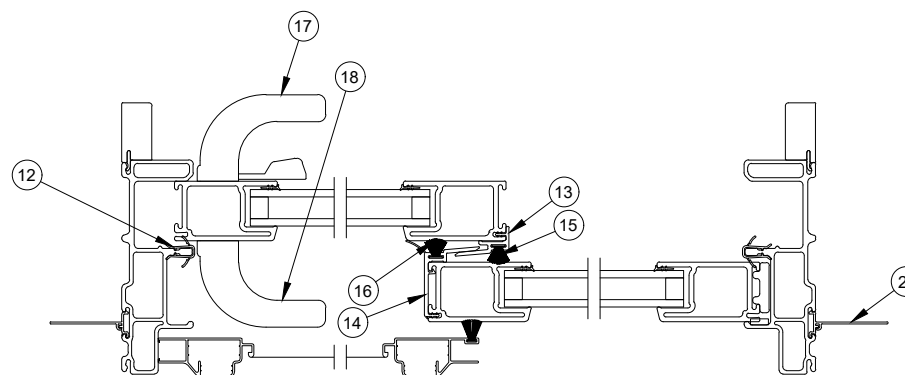
Jamb Detail - 2 Panel XO
