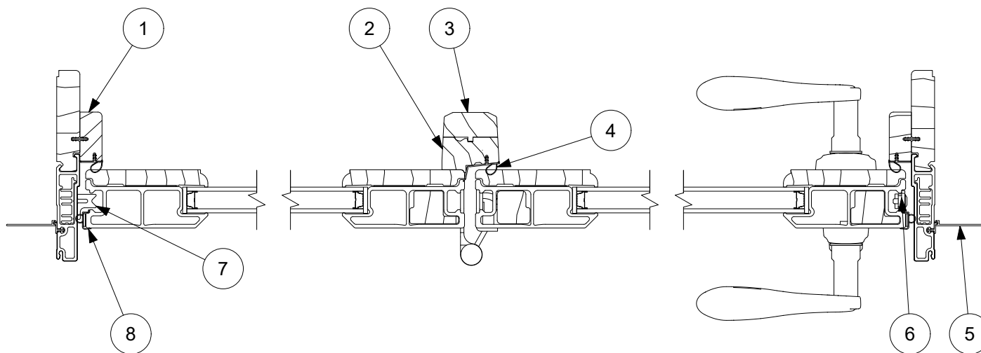
Jamb Detail
