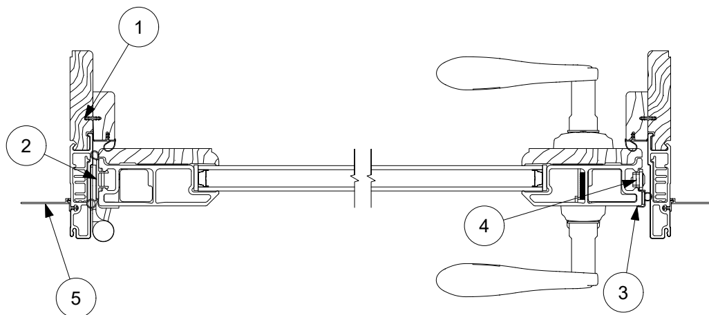
Jamb Detail
