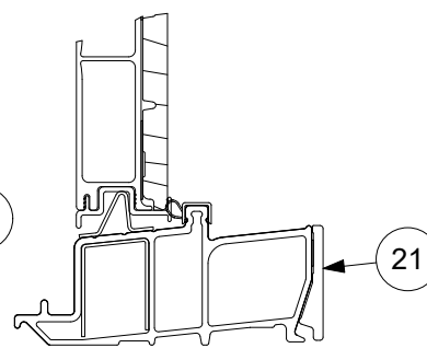
HP/IZ3 Sill Detail
