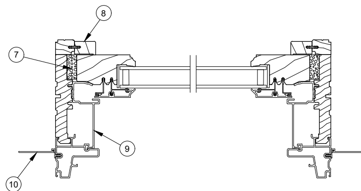
Jamb Detail
