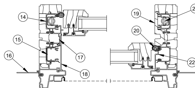
Jamb Details
