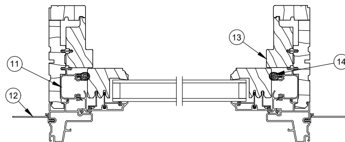
Jamb Detail
