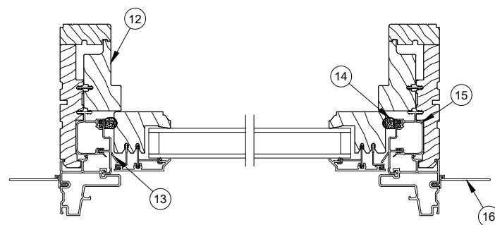
Jamb Detail
