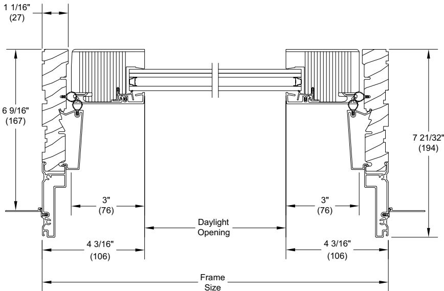
6 9/16" O Jamb
